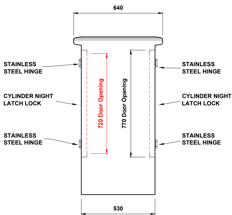
Elevation (C) (l/h side) & Elevation (D) (r/h side)
